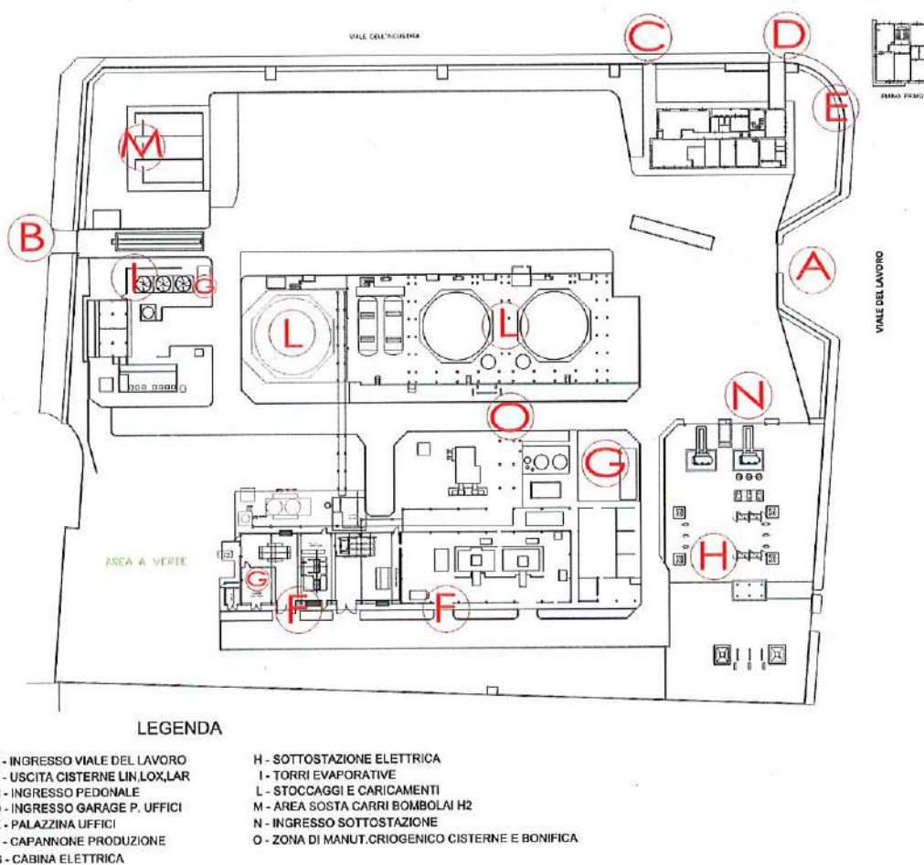
Figura 3: Pianta Stabilimento
