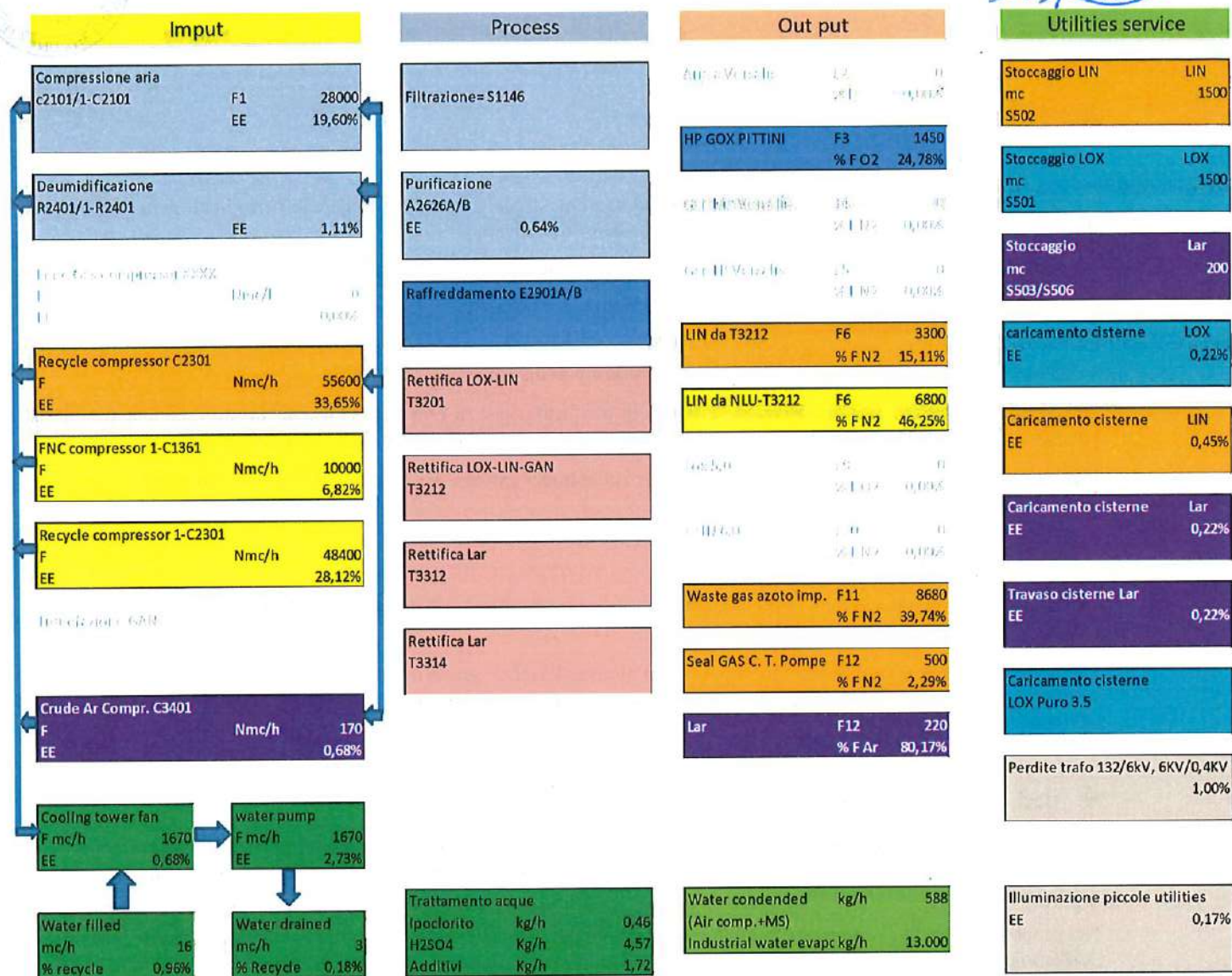
Figura 4: Schema a blocchi dell'impianto
